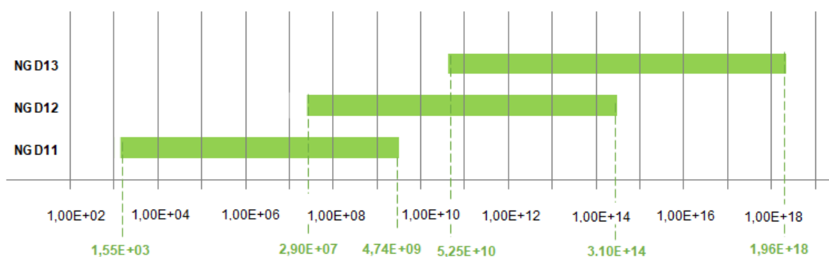
Měřicí rozsahy detektorů NGD-1X ( 85 Kr)
